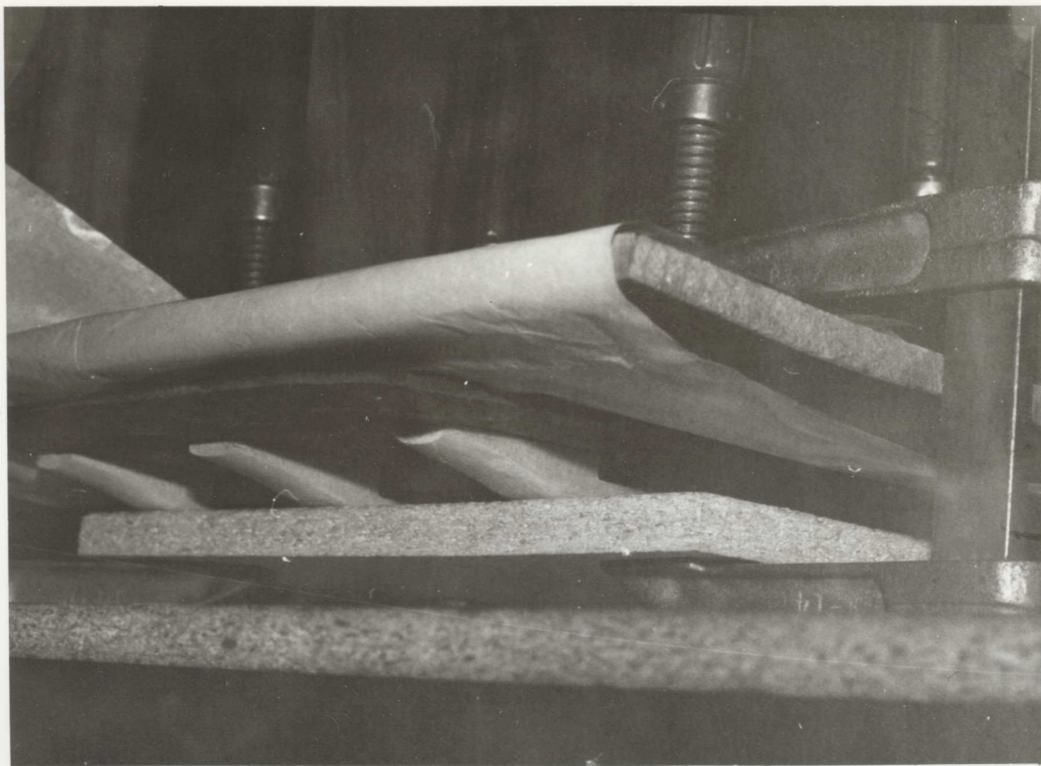
A parkettlécek felragasztása a kiegyenesített táblára.
